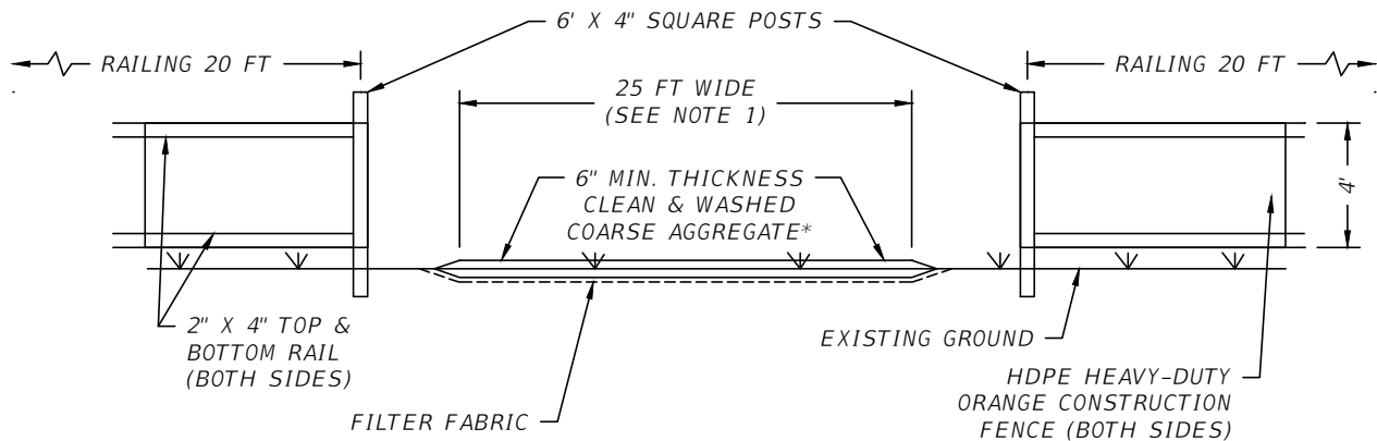
ELEVATION
